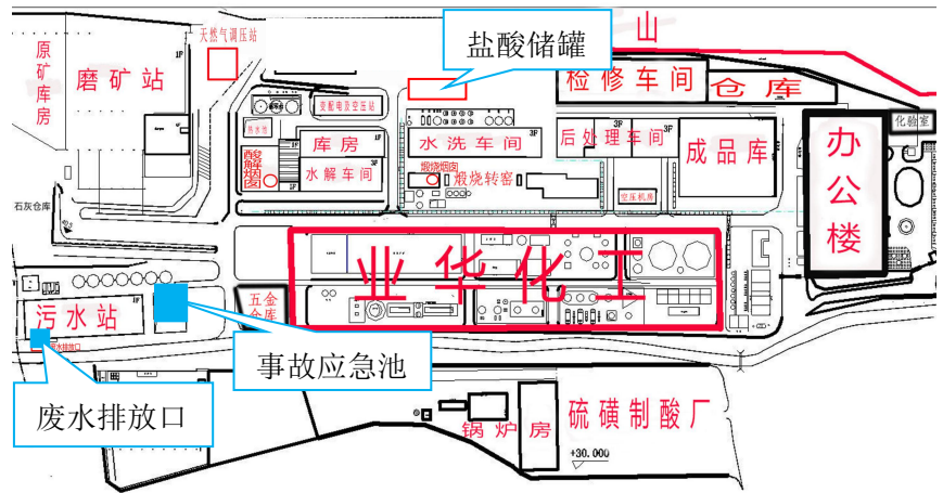
广东惠云钛业股份有限公司钛白二厂厂区平面图
