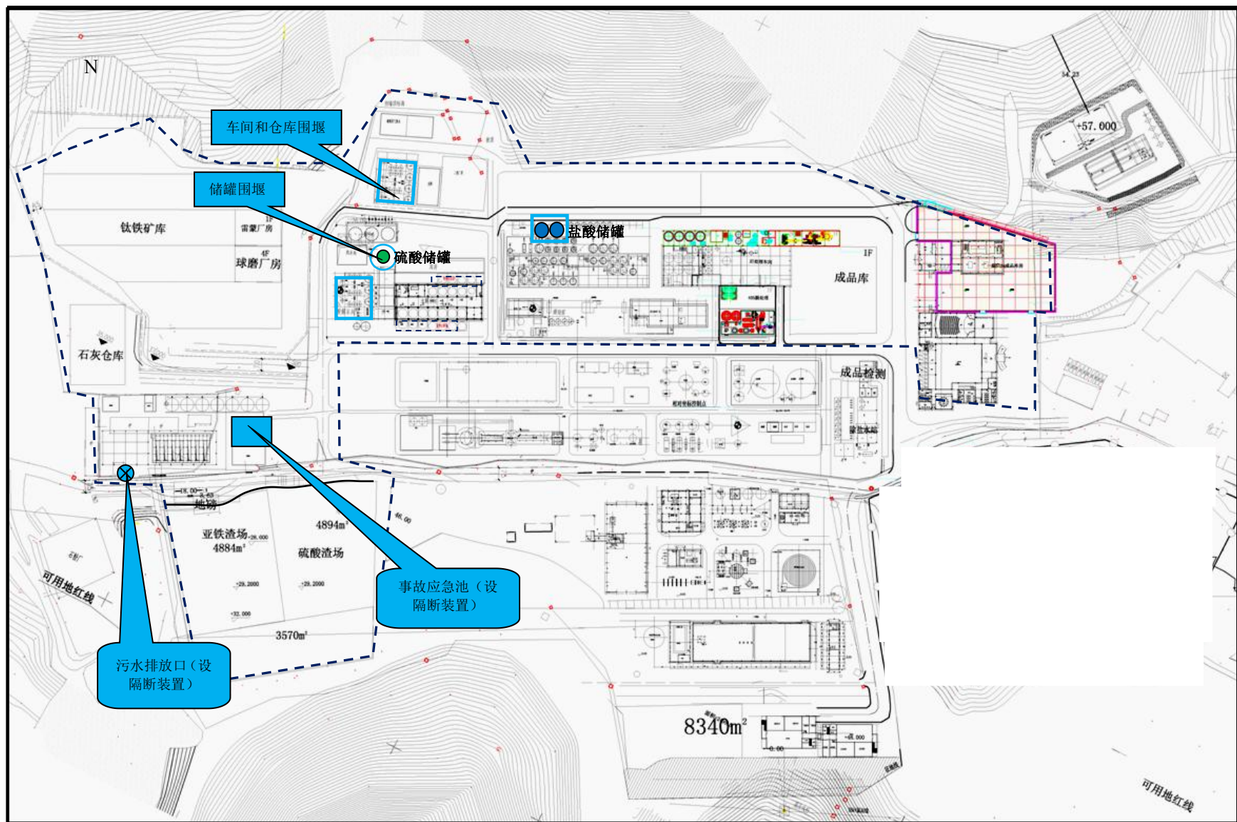
图 7 防止事故废水进入外环境的控制、封堵系统图（厂内）
